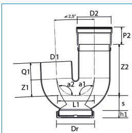
PP+ Sifon met schroefdeksel 1FM
