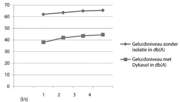
Grafiek 2.1: akoestische eigenschappen Dykasol voorbeeld standleiding 110mm
