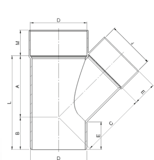
PVC Verloop T-stuk 90x75mm 2 x mof/1 x spie 45°, grijs
