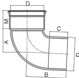
PVC Bocht 90mm mof/spie 90°
