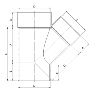
PVC Verloop T-stuk 90x50mm 2 x mof/1 x spie 45°, grijs
