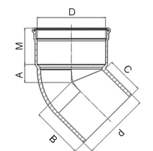
PVC Bocht 90mm mof/spie 45°
