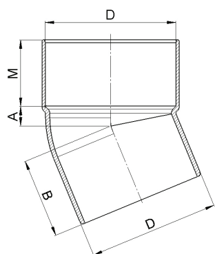
PVC Bocht 90mm mof/spie 45°
