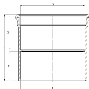
PVC Overgangstuk 2 x mof, grijs
