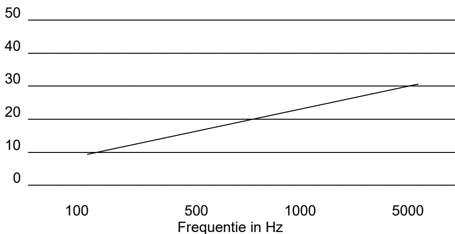
Transmissieverlies volgens ISO R140 Gemiddelde geluidsisolatie-index ca. 20 dB
