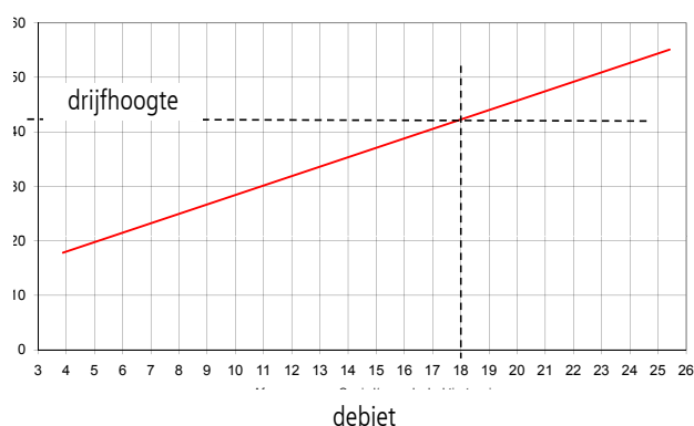
Grafiek 1.3: bij een drijfhoogte van 43 mm is met een 75 mm trechter een afvoercapaciteit van 18 l/s mogelijk.
