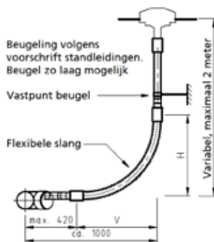
Vooraanzicht
