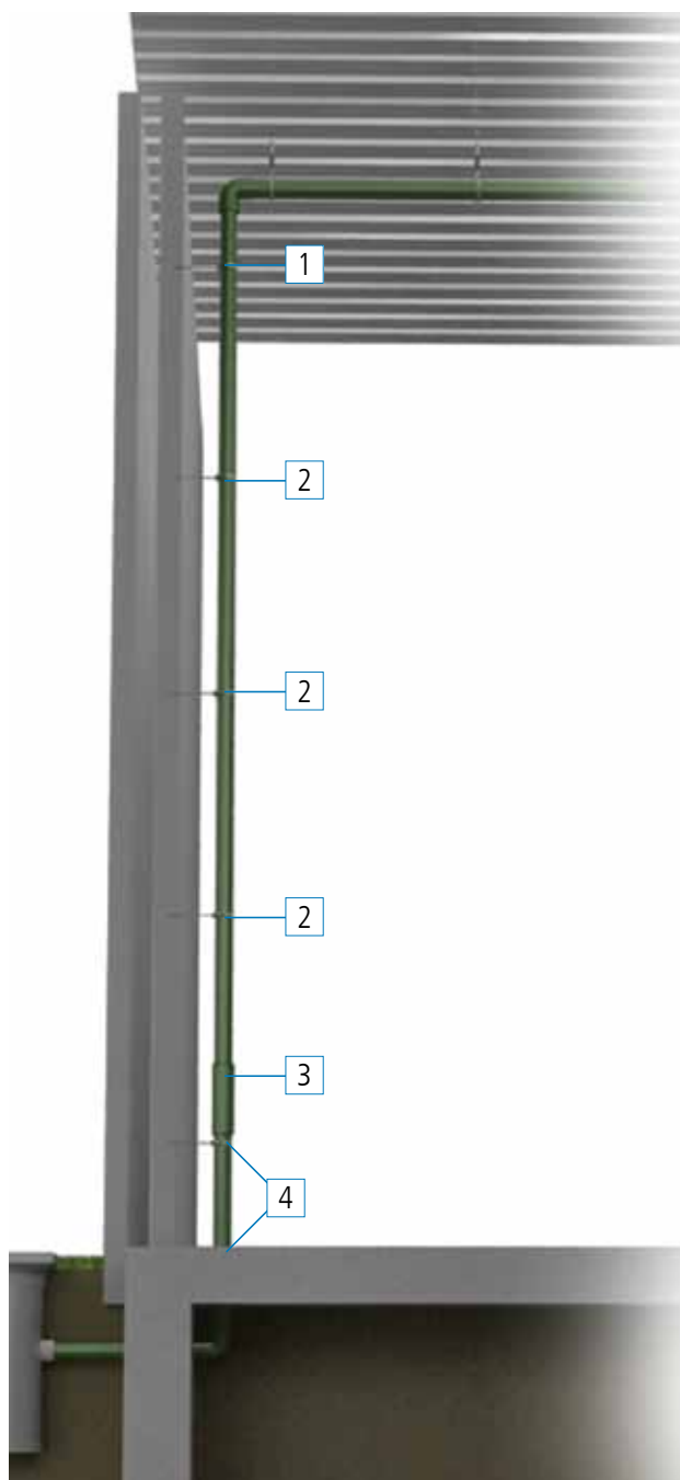
Figuur 4.10: standleiding, vaste punten en expansiestuk
