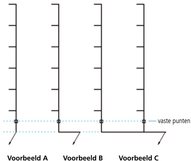
Figuur 4.8: plaats van vaste punten in verzamelleidingen
