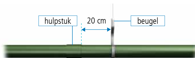
Figuur 4.6: afstand beugel tot hulpstuk minimaal 20 cm
