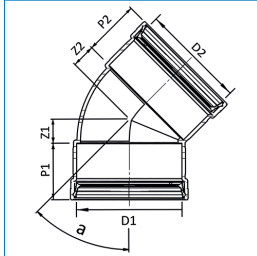
PP+ Bocht 2 x mof 45gr, zwart
