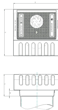
BTN GY Straatkolkkop 315-B125, 334x334
