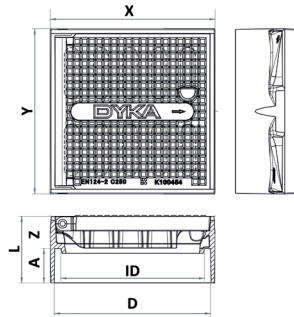
DYKA GY Straatkolkkop SDS 315 C250, blind deksel, vergrendeld
