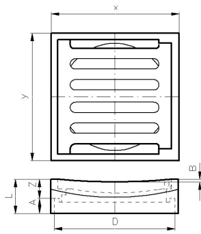
DYKA GY Straatkolkkop SDS 315 C250, vergrendeld
