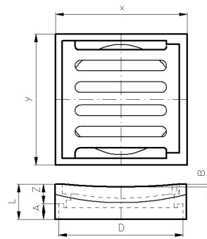
BTN GY Straatkolkkop 315-B125, 334x334, Vergrendeld
