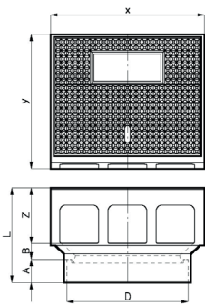
BTN GY Straatkolkkop 315-B125, 350x400, Infiltratie Uitvoering
