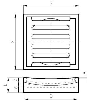
BTN GY Straatkolkkop 315-B125, 334x334, Vergrendeld
