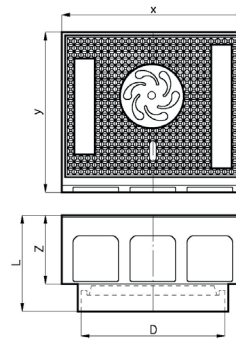
BTN GY Straatkolkkop 315-B125, 450x450, Infiltratie Uitvoering
