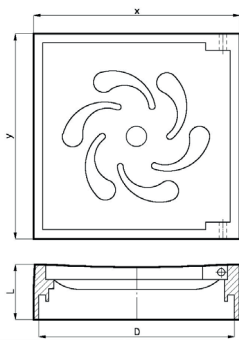
BTN GY Trottoirkolkkop 315-B125 350x400 Infiltratie uitvoering
