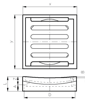
DYKA GY Straatkolkkop SDS 315 C250, laag model
