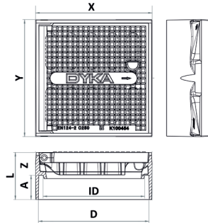
DYKA GY Straatkolkkop SDS 315 C250, blind deksel, vergrendeld
