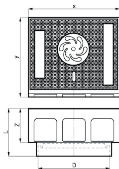
BTN GY Straatkolkkop 315-B125, 350x400, Infiltratie Uitvoering
