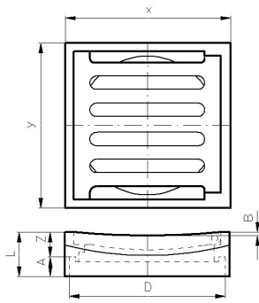
BTN GY Straatkolkkop 315-B125, 334x334, Infiltratie type waaier
