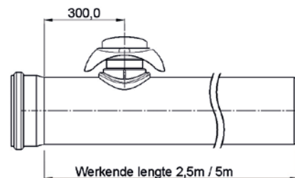
DYKAPrefit Buis met voorgemonteerde inlaat mof/spie
