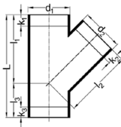
Verloop T-stuk 45°
