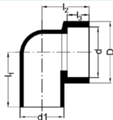
Sifon aansluitbocht 90°
