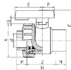
Kogelkranen lijmmof x kraagbus en wartel
