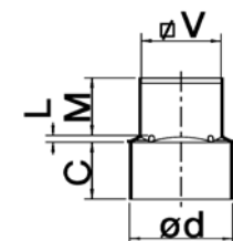
Verloopstukken lijmvverbinding vierkant op rond mof/spie
