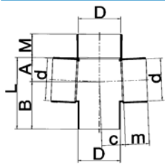
Dubbel T-stuk 87°/30° lijmvverbinding 3x mof/1x spie
