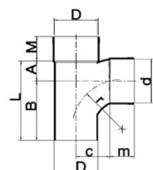
Stroom T-stukken 90° lijmvverbinding 2x mof/1x spie
