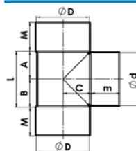
T-stuk 3 x mof 90°
