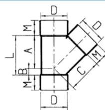
Vacurain T-stukken 45°, 3 x LV
