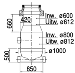
Polyester inspectieput
