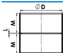
Steekmof 2 x mof
