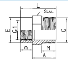
Verloopnippels 1 x buitendraad 1 x binnendraad
