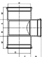
DykaSono T-stuk 3 x mof 87,5°
