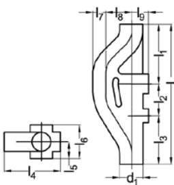
Valleiding/ventilatie T-stuk
