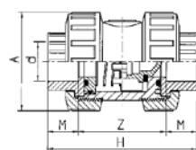
Terugslagkleppen 2 x kraagbus en wartel
