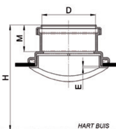
DYKA Prefit inlaat
