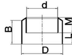
Inzet verloopringen lijmverbinding spie/mof
