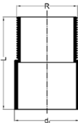
Puntstuk spie/buitendraad
