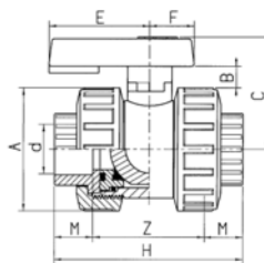
Kogelkranen 2 x kraagbus en wartel
