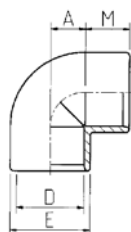
Knieën 90° 2 x lijmmof
