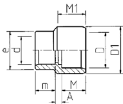
Verloper 1 x lijmmof 1 x spie eind 1 x lijmmof
