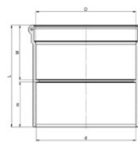
Overgangstuk mof/manchetmof
