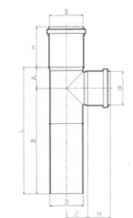
DykaSono Verlengd closet T-stuk 2 x mof/1 x spie 87°
