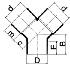
Y-stuk 45° lijmvverbinding 2x mof/1x spie
