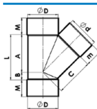
T-stuk 3 x mof 45°
