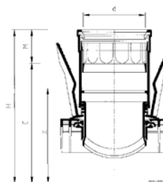
Knevelinlaten met zettingsconstructie
