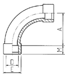
Bochten 90° 2 x lijmmof
