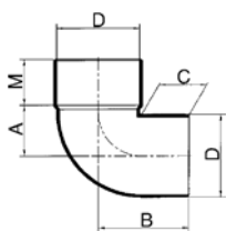
Korte bochten mof/spie 90°
