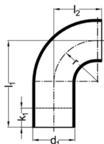
Bocht 90° met lang been
