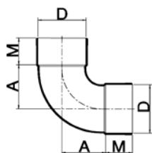
Vacurain bochten 90°, 2 x LV
