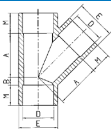
T-stukken 45° 3 x lijmmof
