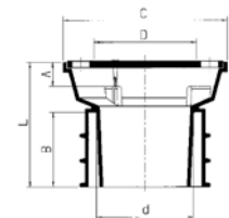
Balkonafvoer
