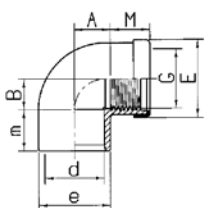
Knieën 90° 1 x lijmmof 1 x binnen dr.
