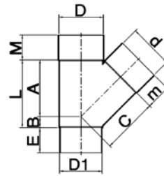
T-stukken 87°30' lijmverbinding 2 x mof/1 x verjongd spie-eind
