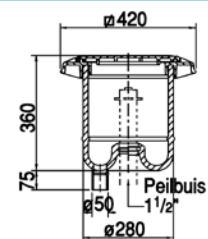
Peilput
