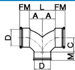
Flexibel stroom T-stuk 90gr manchetverbinding 3x mof Klasse 34 SN 8
