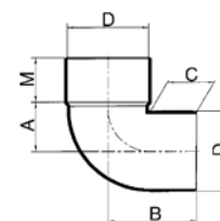
Bocht mof/spie 90°
