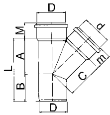
T-stukken 45° manchetverbinding 2 x mof/1 x spie
