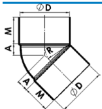
Bocht 2 x mof 45°
