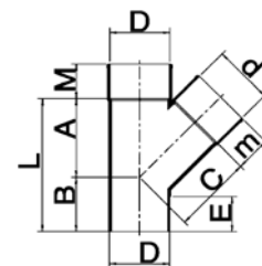
T-stukken 45° lijmverbinding 2 x mof/1 x spie
