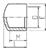
Afsluitkappen lijmmof
