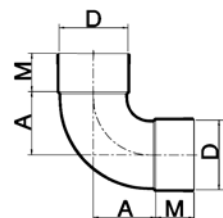
Bochten 90° lijmvverbinding met 2 moffen
