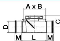
Onstopingsstuk manchetverbinding 2x mof met keerklep Klasse 34 SN 8
