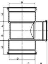
DykaSono Verloop T-stuk 3 x mof 90°
