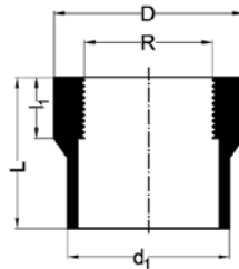
Schroefbus spie/binnendraad
