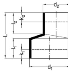
Verloopstuk excentrisch
