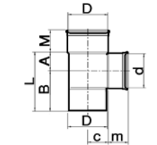
T-stukken 87° 30' manchetverbinding 2 mof 1 spie Klasse 34 SN 8
