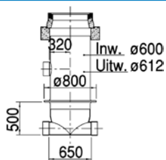
Polyester inspectieput
