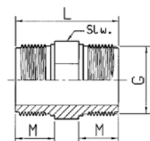
Nippels 2 x buitendraad
