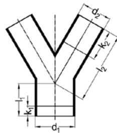
Broek T-stuk 60°
