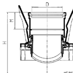
Knevelinlaten zonder zettingsconstructie
