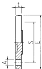
Blindflenzen
