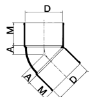
Bochten 45° lijmvverbinding met 2 moffen
