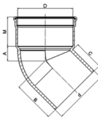
Bocht 45° manchetterverbinding mof/spie
