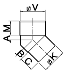
Vierkante bochten 45° lijmvverbinding mof/verjongd spie-eind
