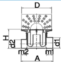
Douchesifon model D15-D en D15-D-R
