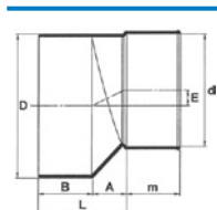
Verloop excentrisch spie/mof
