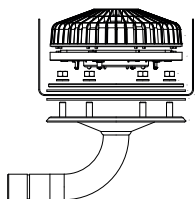
Vacurain flenstrechter 90°
