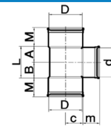
T-stukken 90° manchetverbinding 3 moffen Klasse 34 SN 8
