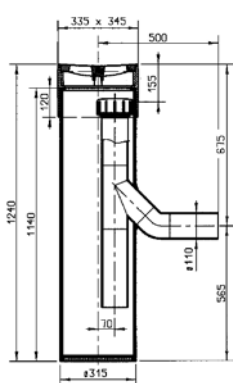
Explosievrije straatkolk PE/GY
