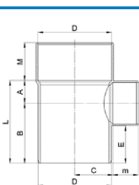
Dubbel T-stuk haaks 90° lijmverbinding met 3 moffen
