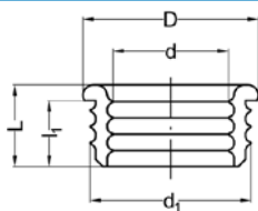
Rubber lippenring voor sifonmof/-bocht
