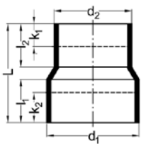
Verloopstuk centrisch
