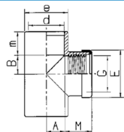
T-stukken 90° 2 x lijmm 1 x binnendraad
