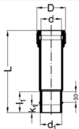
Expansiemof met vastpunt
