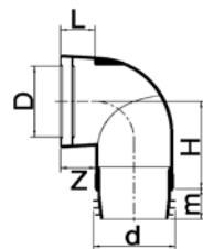
Closetafoerbochten
