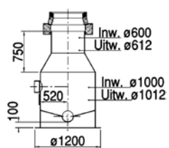
Polyester inspectieput
