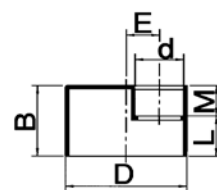
Verloopringen excentrisch lijmvverbinding spie x mof
