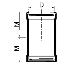
Overschuifmoffen met 2 manchetten
