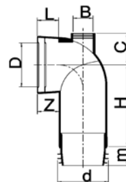
Closetafoerbocht modelnr. 303M
