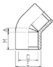
Knieën 45° 2 x lijmmof
