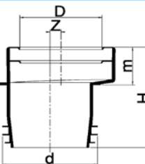
Closetafoermanschiet
