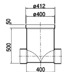
Polyester inspectieput
