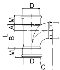
Ontstoppingsstukken met schroefdeksel manchetverbinding met 2 moffen
