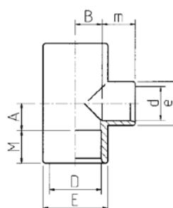
Verloop T-stukken 90° 3 x lijmmof
