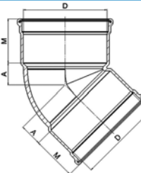
Bocht 45° manchetterverbinding mof/mof
