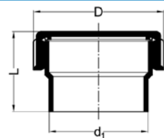
Eindstuk met schroefdeksel lang
