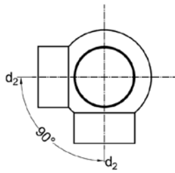
Kogel T-stuk 90°
