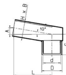
Stadsuitloop 6 x 10 cm (op buis 100)
