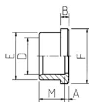
Kraagbussen, vlak lijmmof
