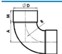
Bocht 2 x mof 90°
