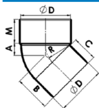
Bocht mof/spie 45°
