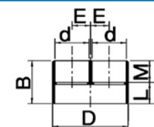
Dubbele verloopringen lijmvverbinding excentrisch spie/mof/mof
