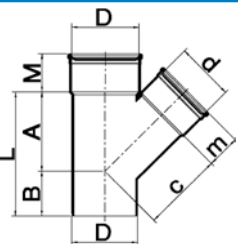
T-stukken 45° manchetverbinding 2 mof 1 spie Klasse 41 SN 4
