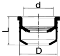
Rubber overgangsrings van metaal op PVC
