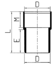
Opzetstukken mof/spie lijmverbinding
