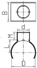
Zadelstukken verlijmbaar
