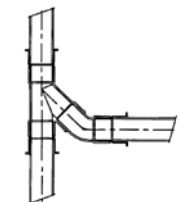
Fixeermof
