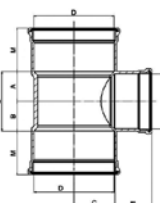
DykaSono T-stuk 3 x mof 90°
