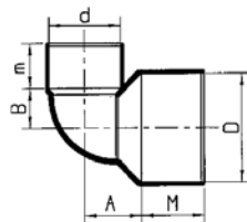
Verloopbochten 90° lijmvverbinding 2 moffen
