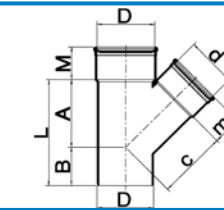
T-stukken 45° manchetverbinding 2 mof 1 spie Klasse 34 SN 8
