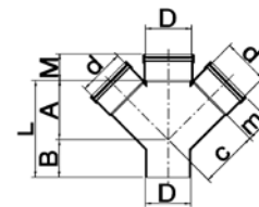
Dubbele T-stukken 90° manchetverbinding 3 mof 1 spie Klasse 41 SN 4
