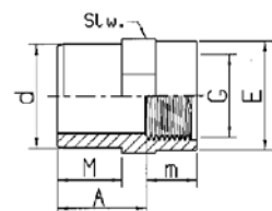
Overgangsspiestukken 1 x spie eind 1 x binnendraad
