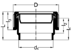
Schroefkoppeling
