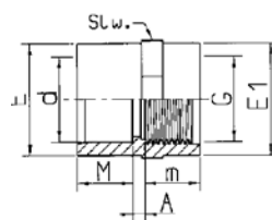
Overgangsmoffen 1 x lijmmof 1 x binnendraad
