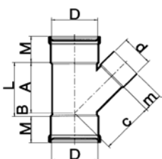
T-stukken 45° met 3 moffen 2x manchiet/1x lijmvverbinding. Doorgaande leiding manchietverbinding aftakking lijmvverbinding.
