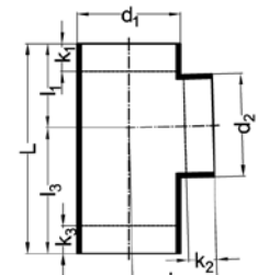
T-stuk 88,5°
