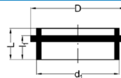
Eindlaskap (40-110 mm)
