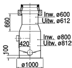
Polyester inspectieput
