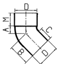
Vacurain bochten 45°, 1 x LV
