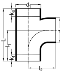
Stroom T-stuk 88,5°
