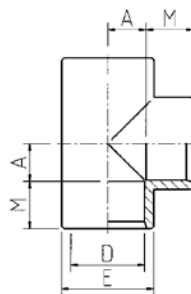
T-stukken 90° 3 x lijmmof
