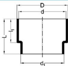
Vloerclosetmof
