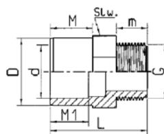
Verloopmoffen 1 x lijmmof 1 x spie eind 1 x buitendraad
