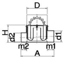
Douchesifon model D10-D en D10-D-R
