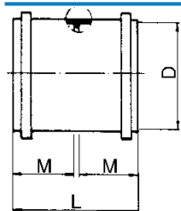
Expansie Steekmof 2 x mof
