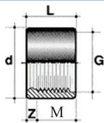
Verloperingen 1 x spie eind 1 x binnendraad
