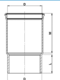
DykaSono inbouw mof mof/spie
