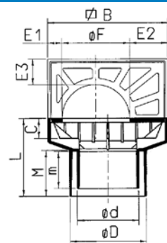
Ontlastputten
