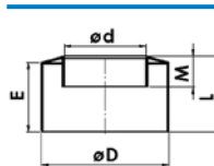
Inzetverloopring centrisch spie/mof
