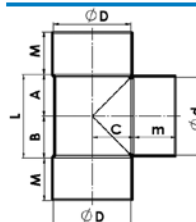
Verloop T-stuk 3 x mof 90°
