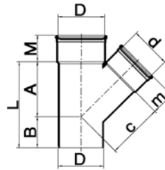
Verloop T-stukken 45° manchetverbinding 2 mof 1 spie Klasse 41 SN 4
