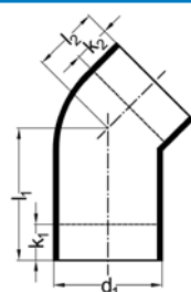
Bocht 45° met lang been
