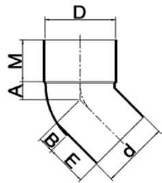
Bochten 45° lijmverbinding mof/verjongd spie-eind
