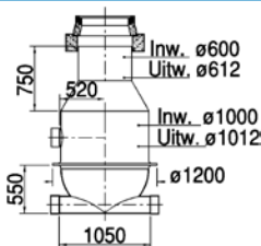
Polyester inspectieput
