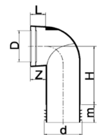
Closetafoerbocht
