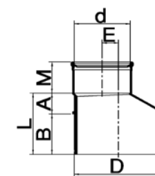
Verloopstukken manchetverbinding mof/spie Klasse 34 SN 8
