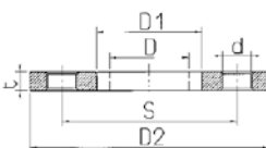
Flens, staal epoxy gecoat
