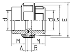
Driedelige koppelingen 2 x lijmmof
