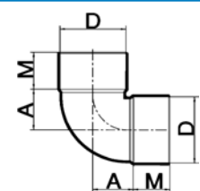
Korte bochten 90° lijmvverbinding met 2 moffen
