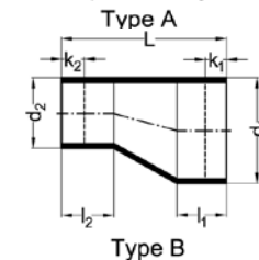
Verloopstuk excentrisch lang type B
