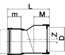
Flexibel huis-kolkaansluitingen manchetterverbinding
