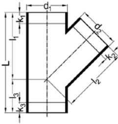
T-stuk 45°
